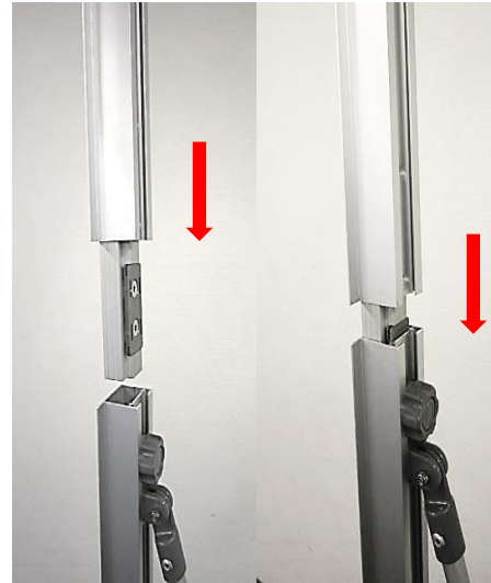
③延伸パーツを本体のアルミフレームに差 し込む。
