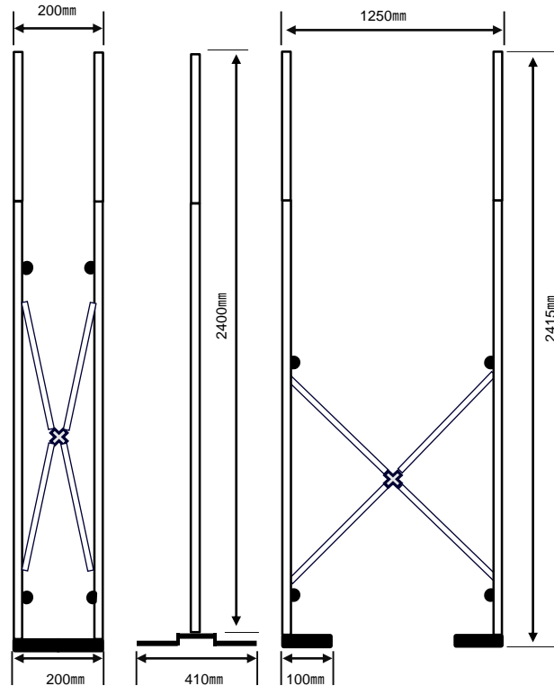
延伸パーツ取り付け後の寸法図
