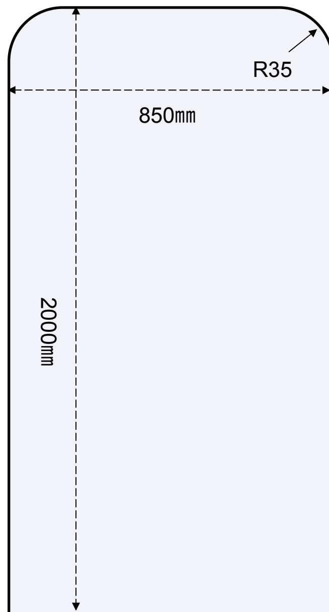
②伸縮ファブリック(布生地)幕サイズ: W850mm × H2000mm パイプ直径: Φ25mm
