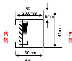
アルミフレームの断面図
