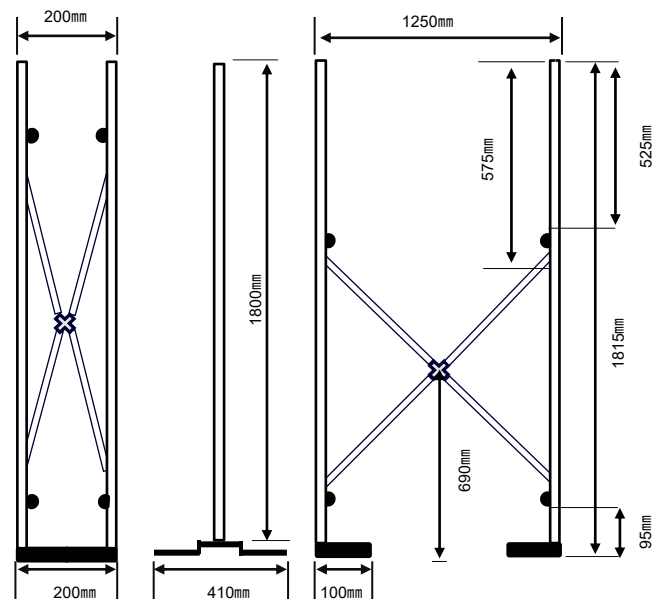
寸法図
