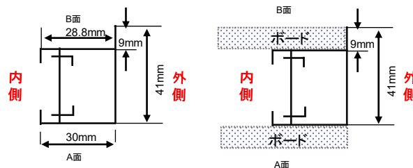
アルミフレームの断面図
